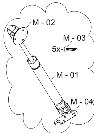
M- Pistão a gás 60N cinza força invertida (1X) Cod 54099
