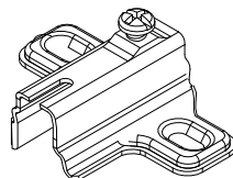
J- Calço H12 p/dobradiça 26mm (2X) Cod 54980
