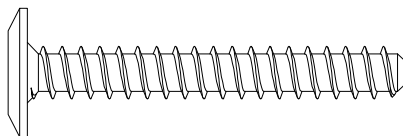
H- Parafuso estrutural ZP 7,0X50mm sx interno cab 17mm (4X) Cod 15892
