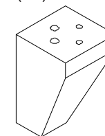
W- Pé madeira Sol (4x) Cod 61239
