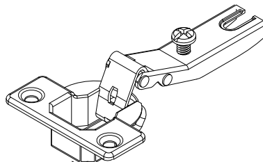
I- Dobradiça SB 26 mm calço 5 (2X) Cod 3826
