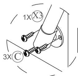
Detalhe (B)
