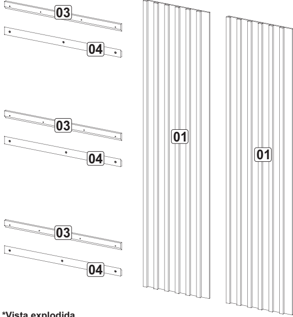
*Vista explodida
