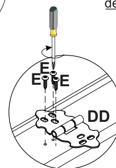
detalhe 14
