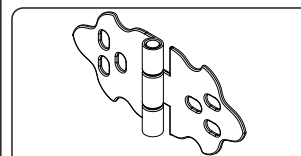
DD- Dobradiça 62mm OV 07.05.202 (BIGFER) (4x)
