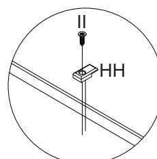
detalhe 29
