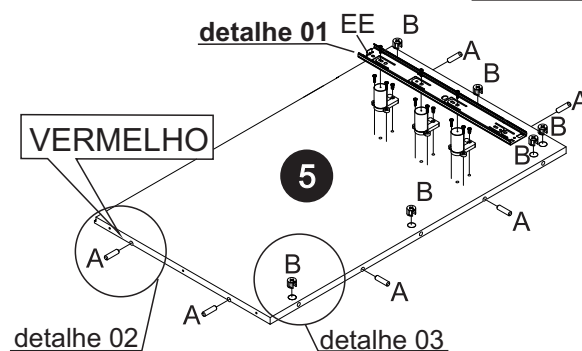
detalhe 03
