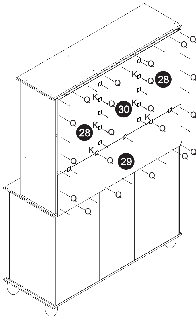
detalhe 10
