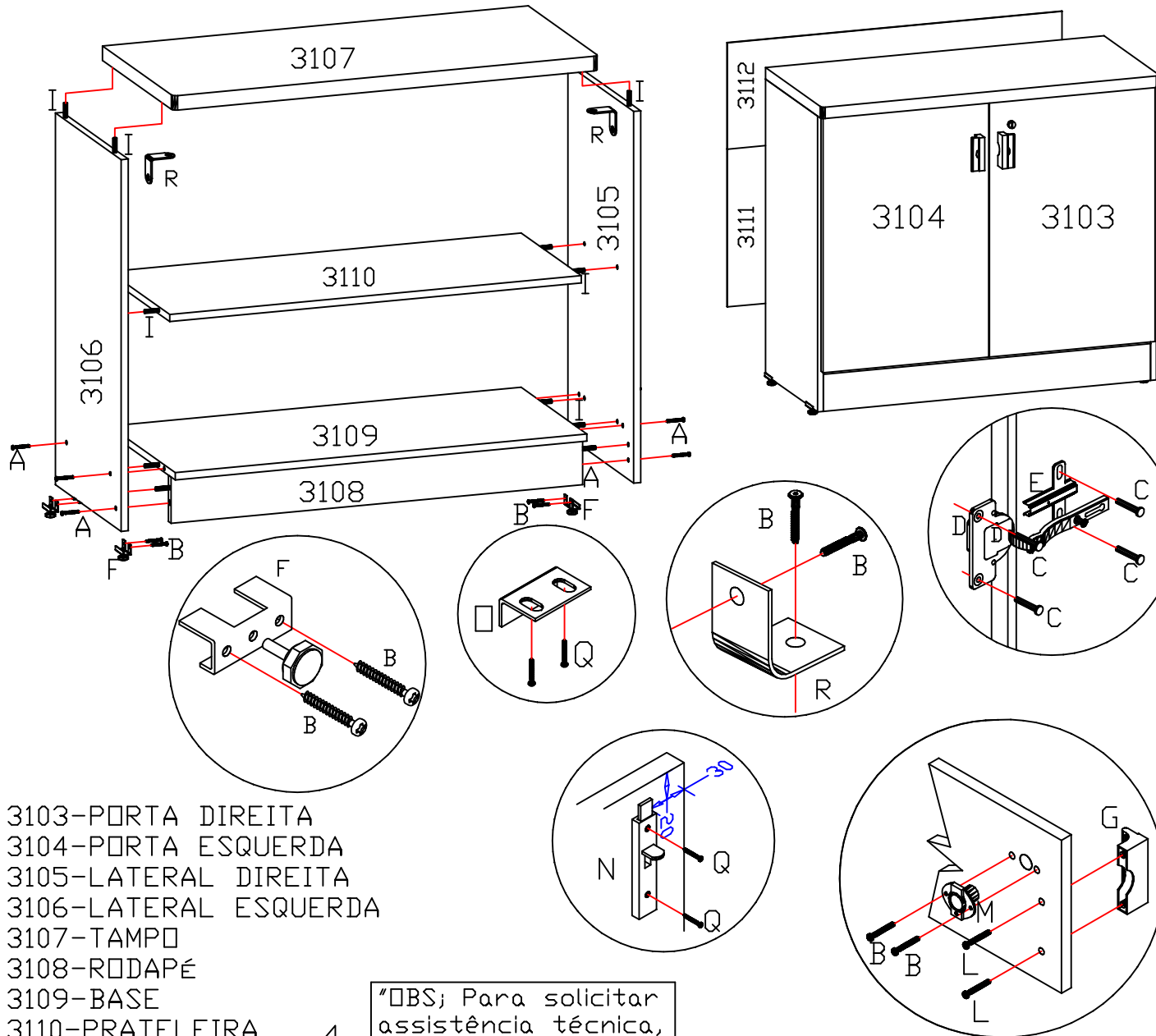
DETALHE DE COMO FIXAR O PUXADOR E A FECHADURA.
