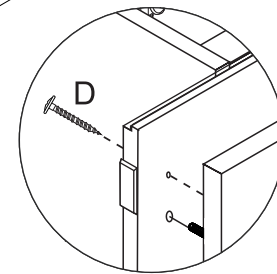
Detalhe 9
