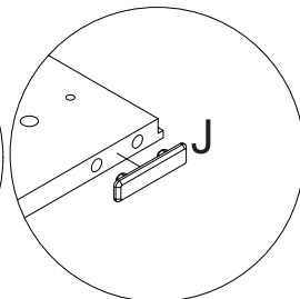
Detalhe 4
