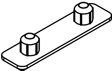
J- Sapata Deslizadora Branca 2 Pinos Chapa 15mm (4x) Cod 2891
