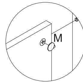
Detalhe 8
