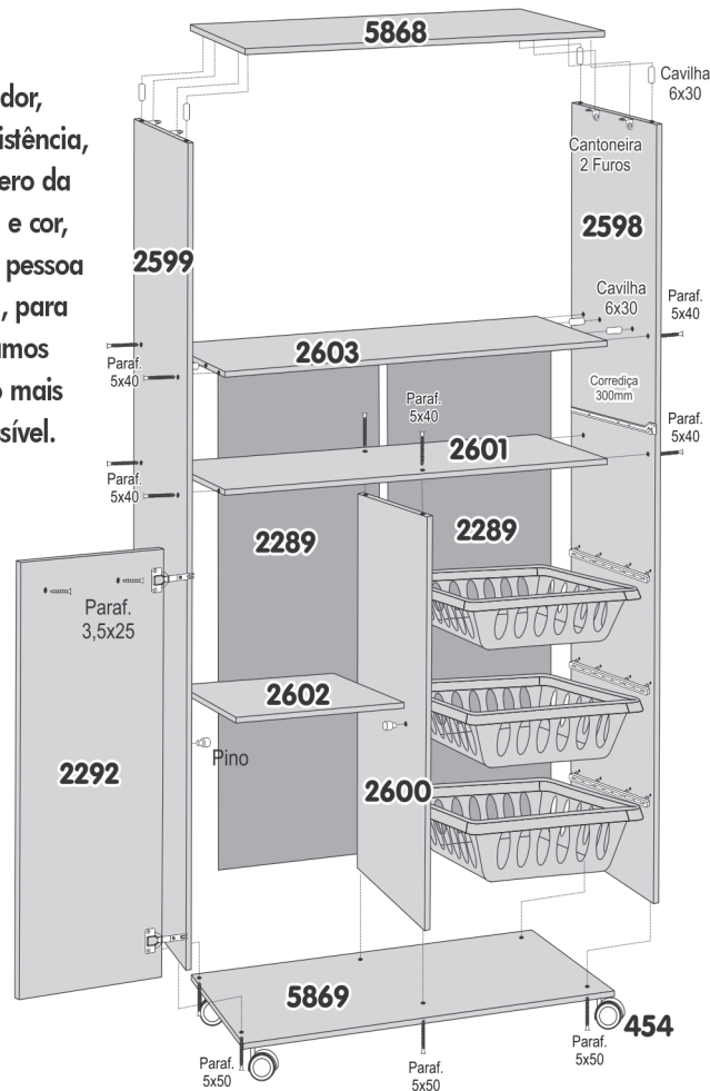
8 - CAVILHA 6x30
