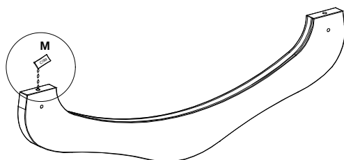
Detalhe da aplicação de cola nas furações.
