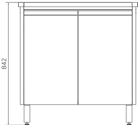
Vista Frontal (mm)
