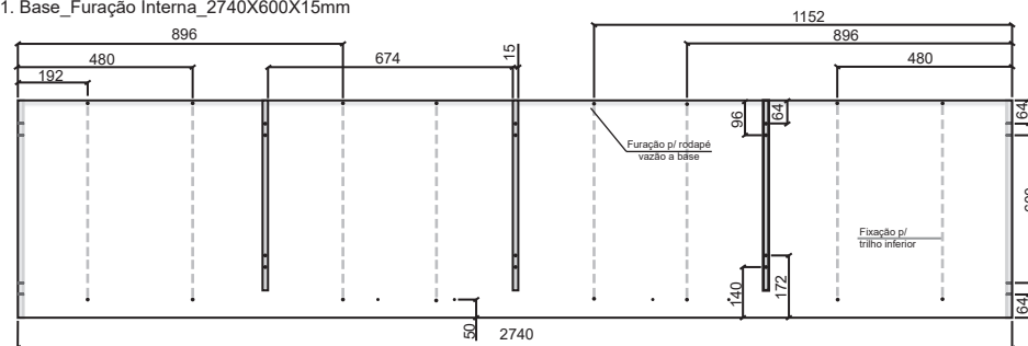
1. Base_Furação Interna_2740X600X15mm
