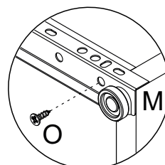
Detalhe 11 Detail/Detalle
