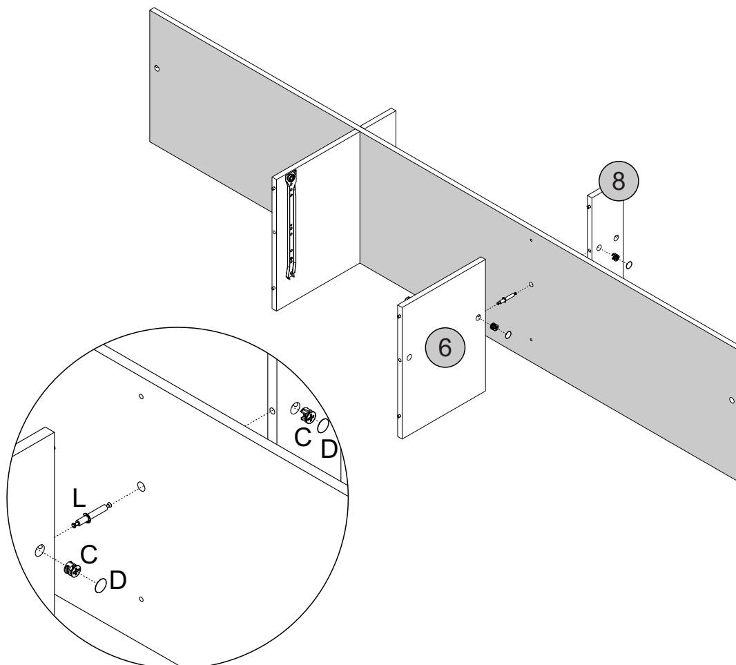
Detalhe 6
