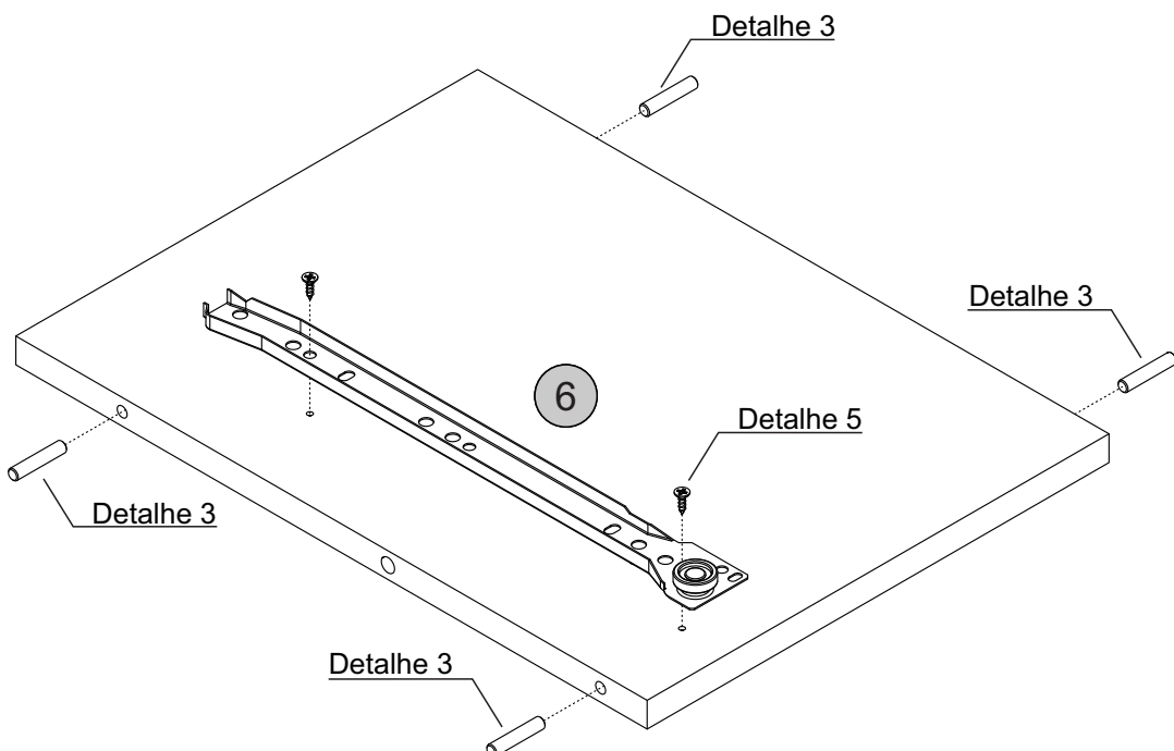
Detalhe 3 Detail/Detalle
