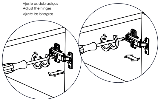
DETALHE B
