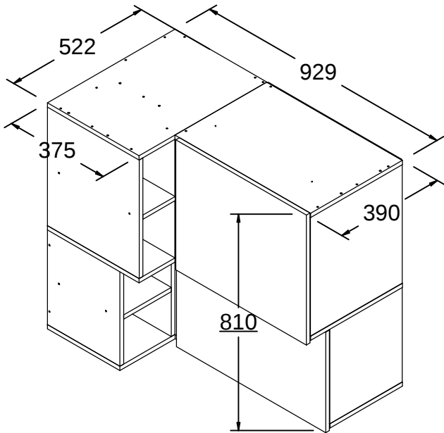
MONTAGEM DO LADO DIREITO. MONTAJE DEL LADO DERECHO. RIGHT SIDE ASSEMBLY.
