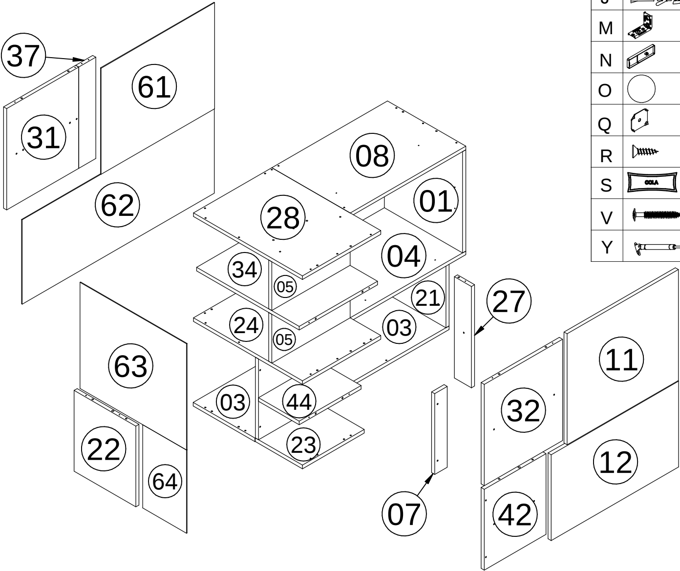
MONTAGEM DO LADO ESQUERDO. MONTAJE DEL LADO IZQUIERDO. LEFT SIDE ASSEMBLY.
