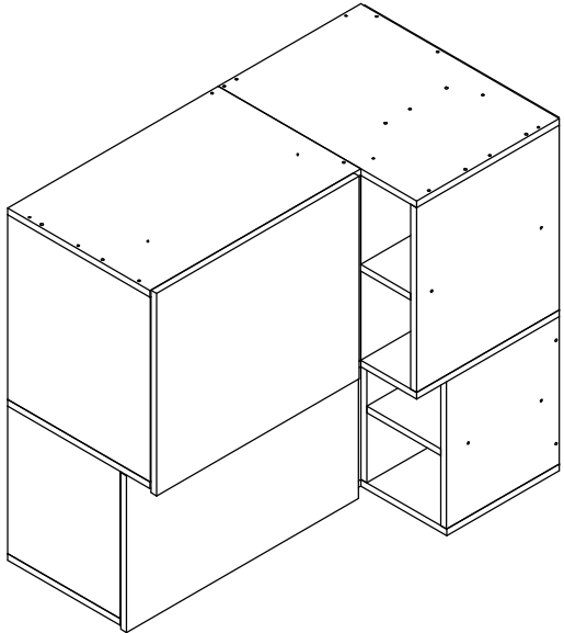
MONTAGEM DO LADO ESQUERDO. MONTAJE DEL LADO IZQUIERDO. LEFT SIDE ASSEMBLY.
