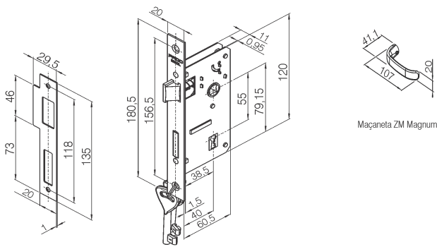
Máquina 30l e contra testa
