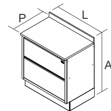
BALC 1PH1G-80 PRODUTO MONTADO: A: 925 L: 801 P: 530 MM
