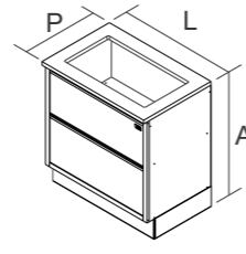
BALC 1PH1G COOK 5B-80 PRODUTO MONTADO: A: 855 L: 801 P: 530 MM
