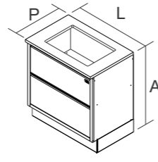
BALC 1PH1G COOK 4B-80 PRODUTO MONTADO: A: 855 L: 801 P: 530 MM
