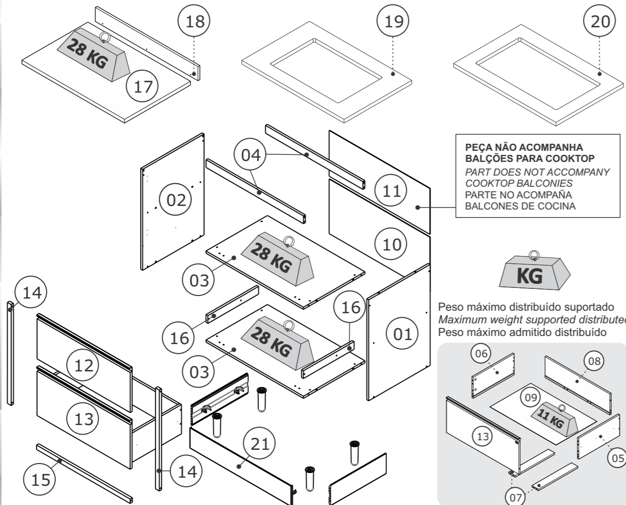
BALC 1PH1G-80 PRODUTO MONTADO: A: 925 L: 801 P: 530 MM
