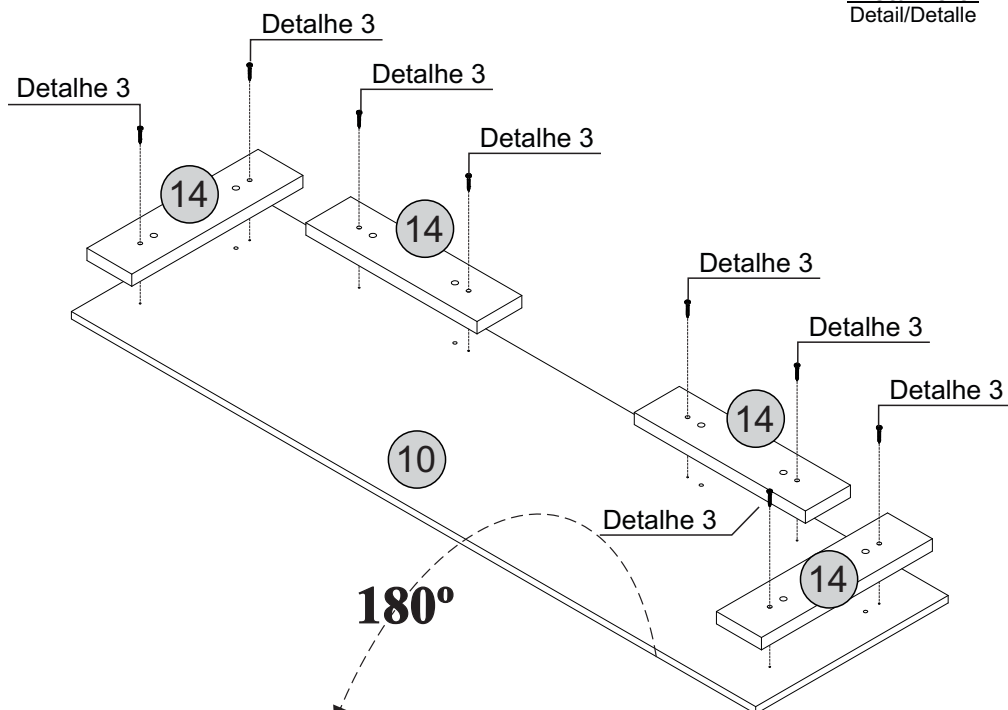
Detalhe 3 Detail/Detalle
