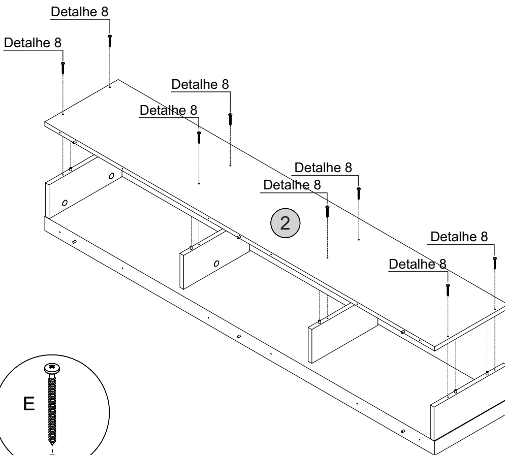
Detalhe 8 Detail/Detalle
