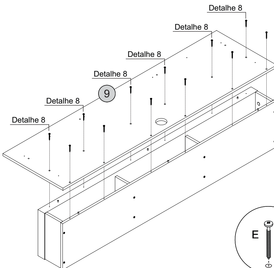
Detalhe 8 Detail/Detalle
