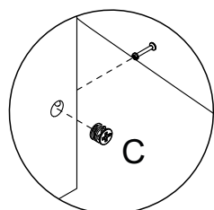
Detalhe 4 Detail/Detalle
