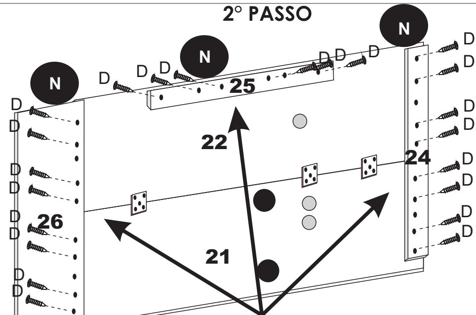
VISTA TRASEIRA
