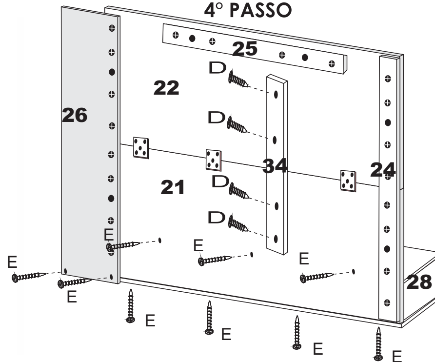
VISTA TRASEIRA
