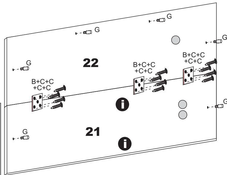
VISTA TRASEIRA
