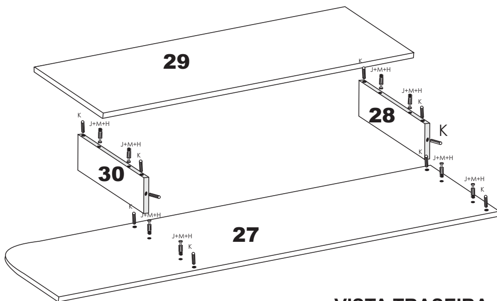
VISTA TRASEIRA
