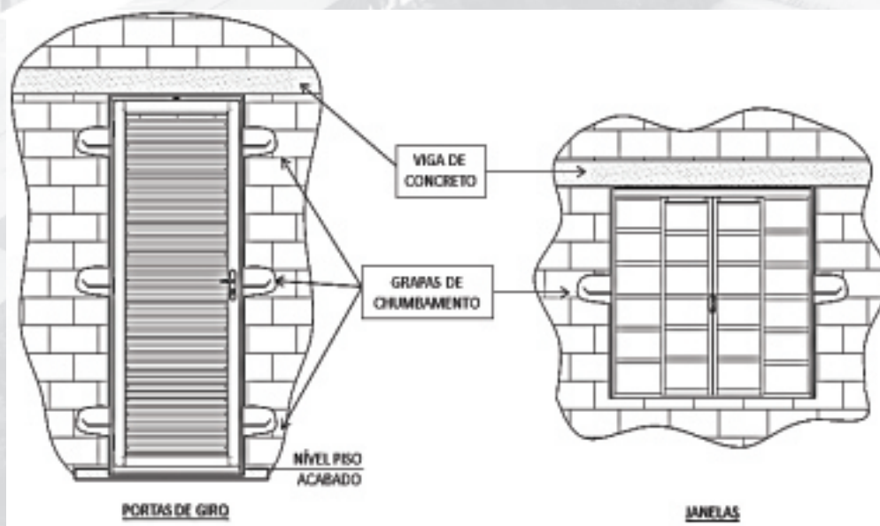
Figura 2 – Descritivo de chumbamento por grapas
