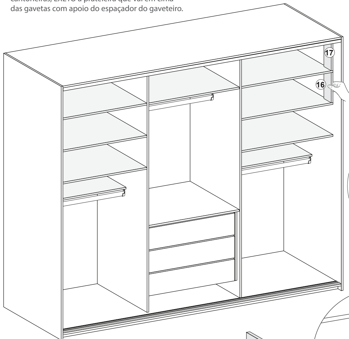
Fig.16 Gabarito P/ prateleira 70x250 mm Fig.17 Gabarito P/ prateleira 70x300 mm
