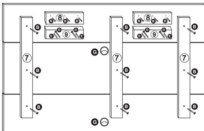
Vista traseira
