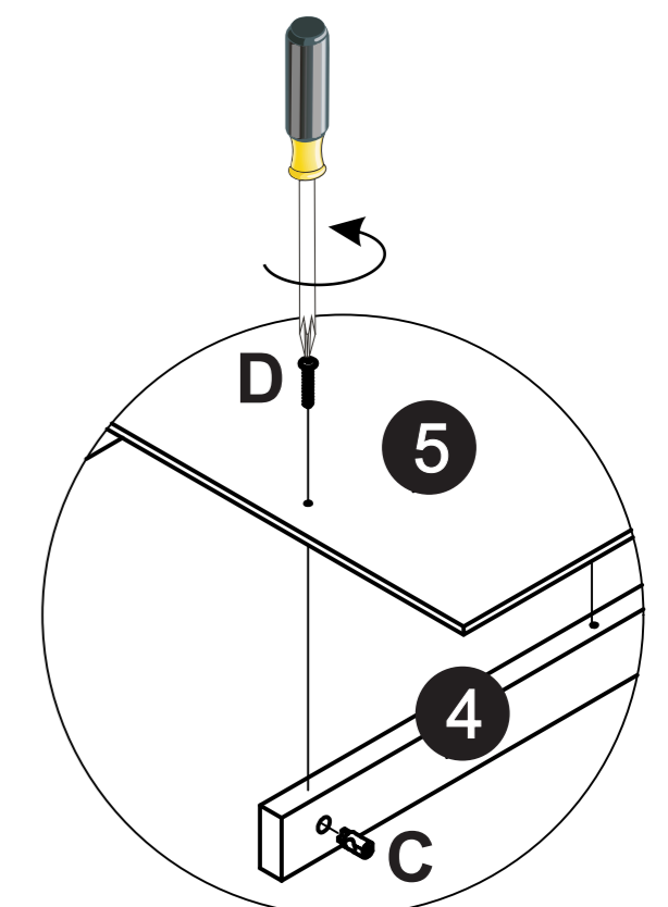
detalhe 02
