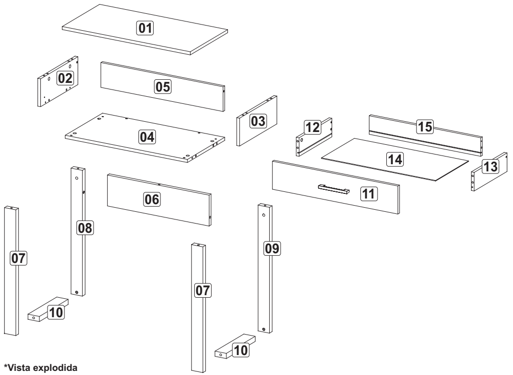
*Vista explodida
