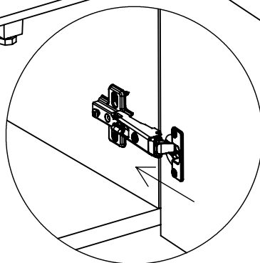
DETALHE A
