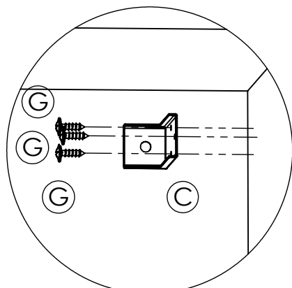
DETALHE A ESCALA 1 : 3
