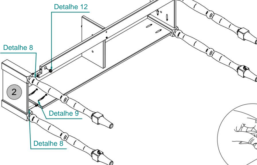
Detalhe 8
