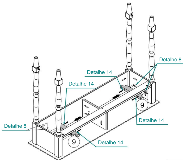
Detalhe 8
