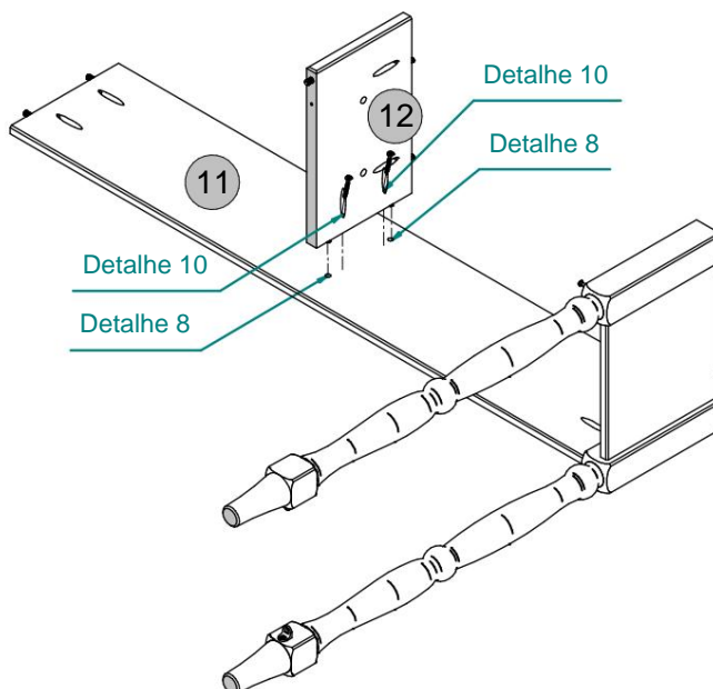
Detalhe 9
