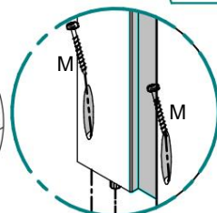
Detalhe 19
