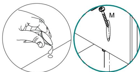
Detalhe 8
