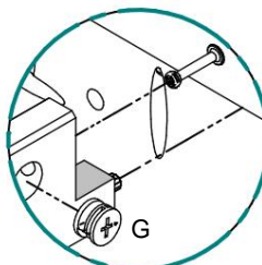
Detalhe 12
