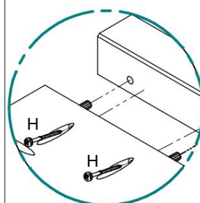
Detalhe 7
