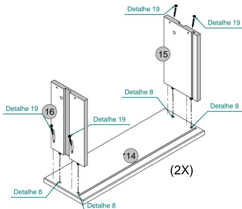
Detalhe 1
