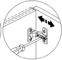
Regulagem Profundidade
