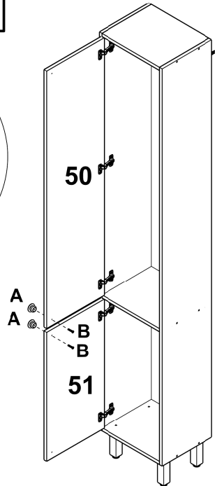
Regulagem Profundidade
