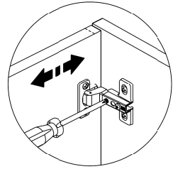
Regulagem Horizontal
