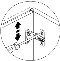
Regulagem Vertical
