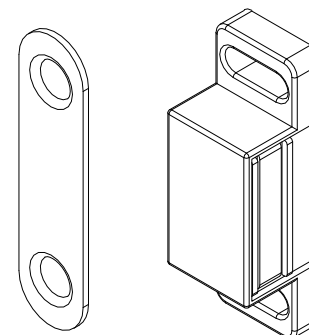
U- Fecho Magnético (SOPRANO) (2x) Cod 333
