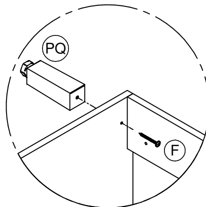
Detalhe A
