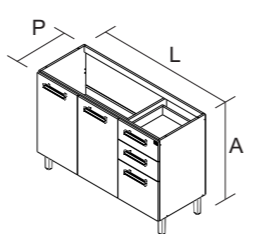
BALC 3PT 2GV ST 120 PRODUTO MONTADO: A: 851 L: 1201 P: 470 MM
