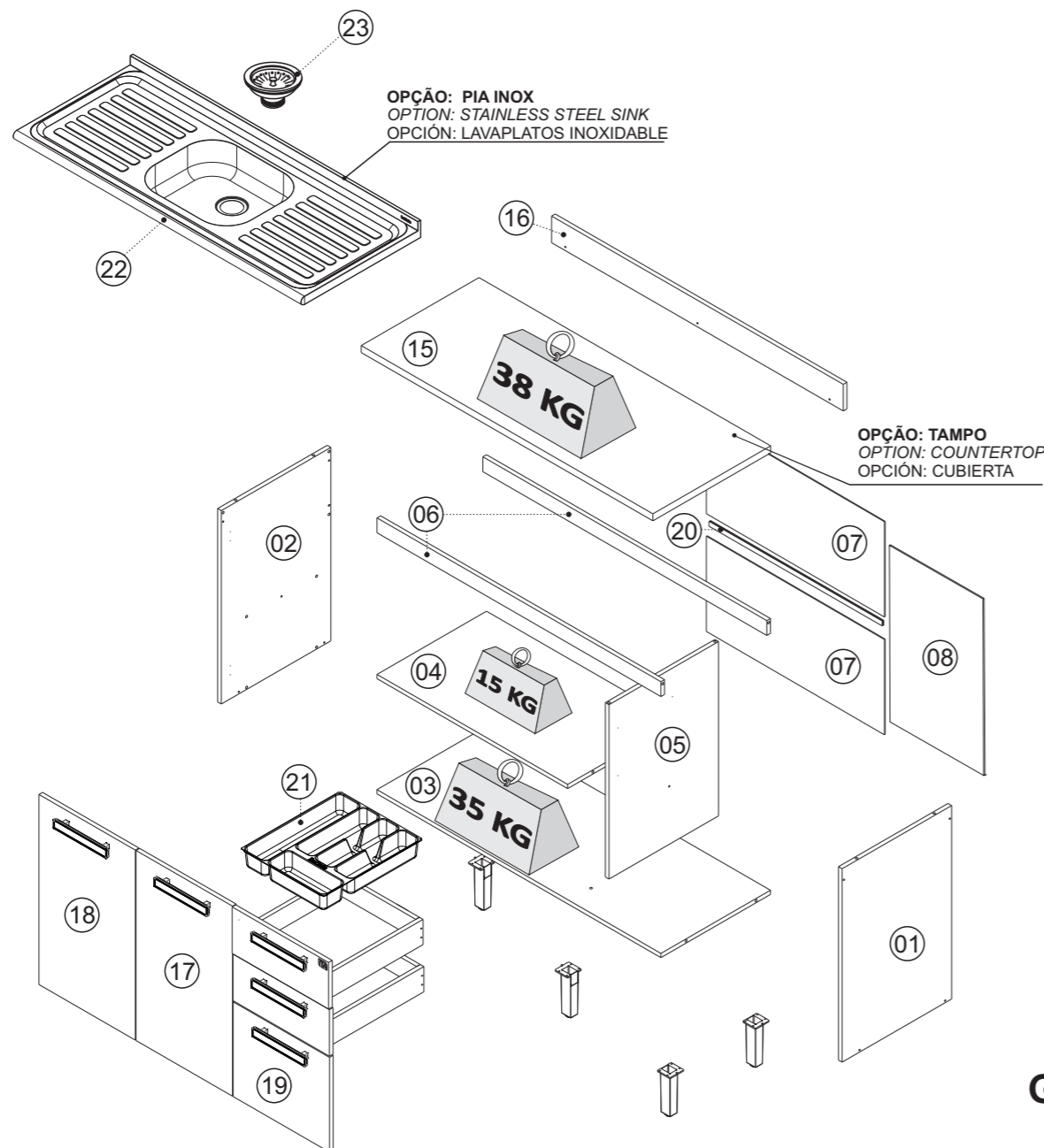
BALC 3PT 2GV 120 PRODUTO MONTADO: A: 921 L: 1201 P: 500 MM
