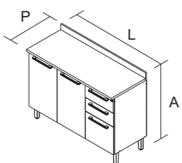
BALC 3PT 2GV 120 PRODUTO MONTADO: A: 921 L: 1201 P: 500 MM
