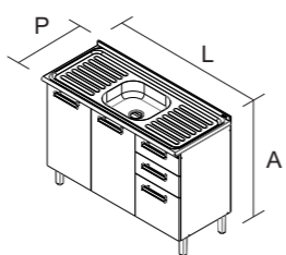
BALC 3PT 2GV PIA 120 PRODUTO MONTADO: A: 914 L: 1201 P: 520 MM
