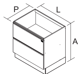
BALC 1PH1G-80 ST PRODUTO MONTADO: A: 830 L: 800 P: 585 MM
