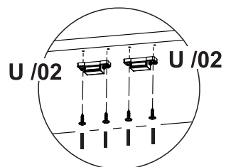
detalhe 11
