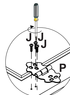
detalhe 16
