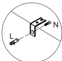
detalhe 6/detalle 6
