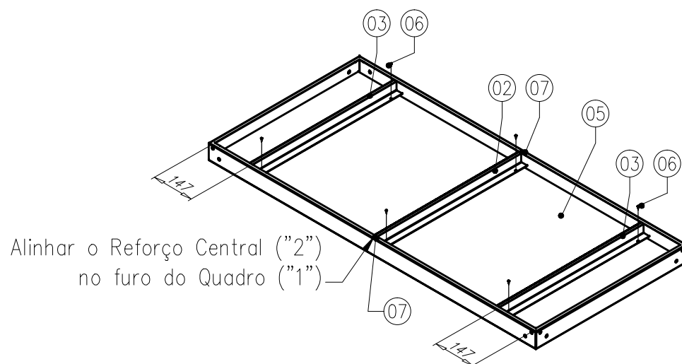
Detalhe Inferior Tampo Esc.: S/E
