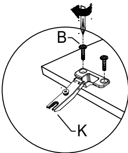
Detalhe 3 detail 3 / detalhe 3
