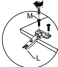
Detalhe 5 detail 5 / detalhe 5
