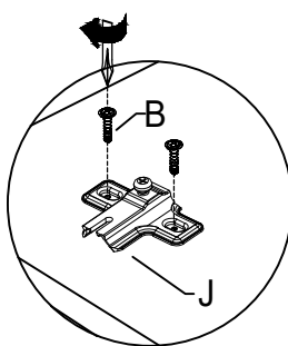
Detalhe 4 detail 4 / detalhe 4
