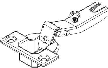
I- Dobradiça SB 26 mm calço 5 (6X) Cod 3826
