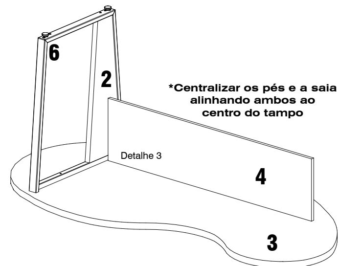
Passo 2
