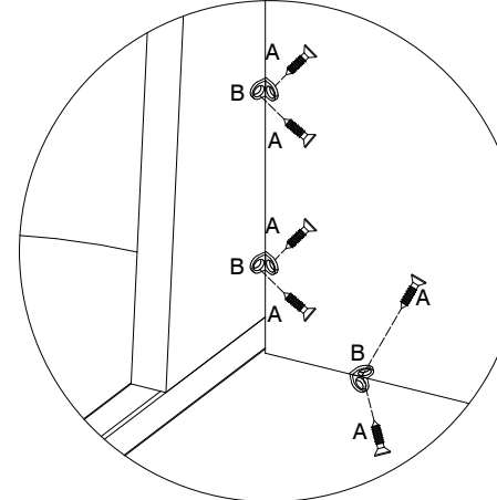
Detalhe 3
