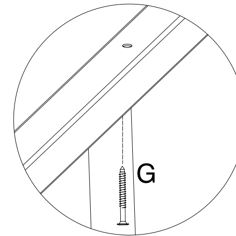
Detalhe 2
