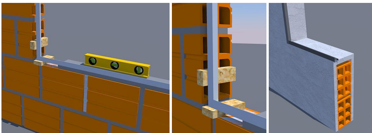
Figura 5 – Assentamento por contramarco
