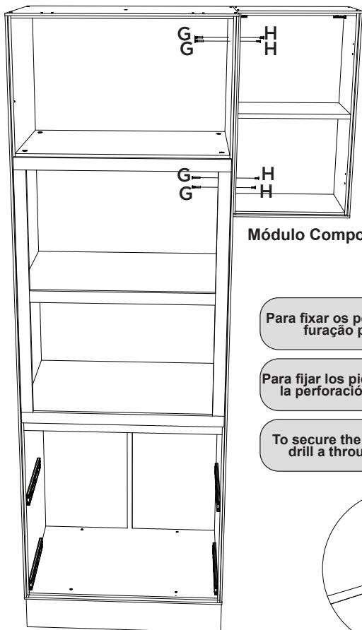
Torre Quente 2 Fornos
