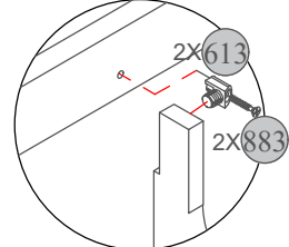
Detalhe (C)
