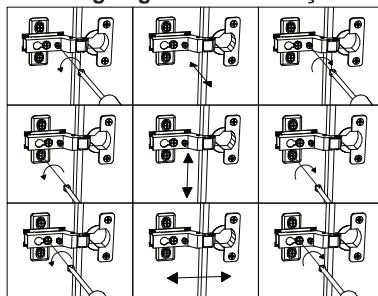
Regulagem da Dobradiça
