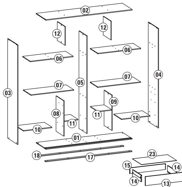
Partes da Porta Parte de la Puerta Door parts
