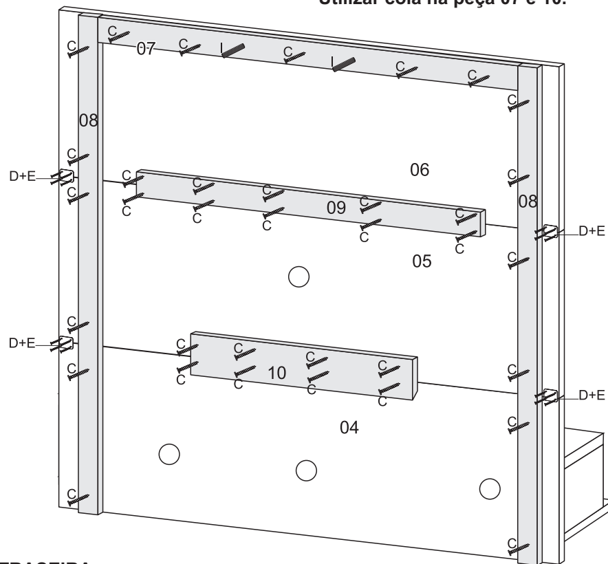
VISTA TRASEIRA
