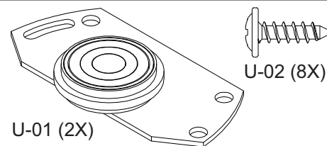
U- Kit sistema correr 1 porta cm 50 - guia silence 25,5 11901 (2X)
