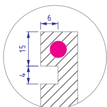
Peça 12 com canal
