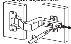
AJUSTE DE PROFUNDIDADE Ajuste de profundidad Depth adjustment
