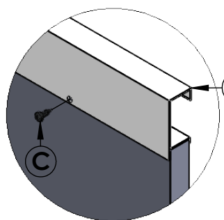
Montagem Puxador
