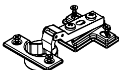
i DOBRADIÇA 6
