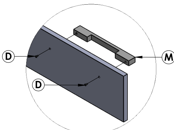
Montagem Puxador Alça
