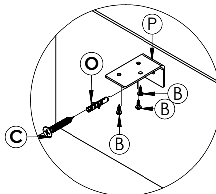
Fixação na Parede
