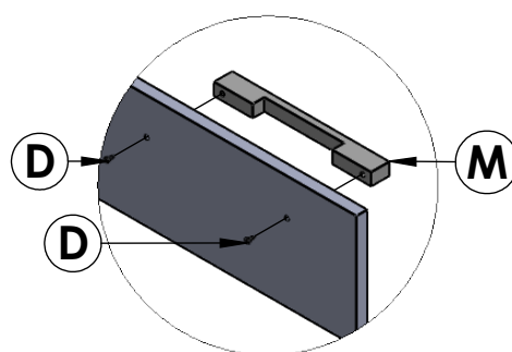
Montagem Puxador Alça
