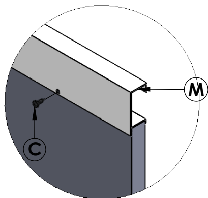
Fixação Puxador Gola
