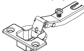
J- Dobradiça SB 26 mm calço 5 (4X) Cod 3826
