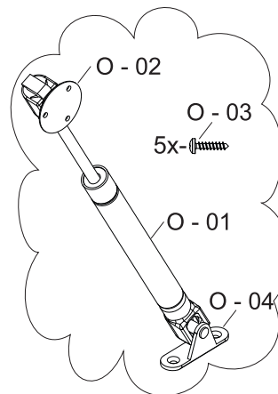
O- Pistão a gás 60N cinza força invertida (2X) Cod 54099
