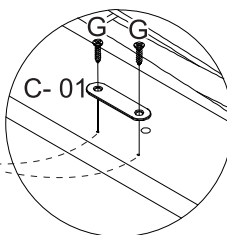
detalhe 13
