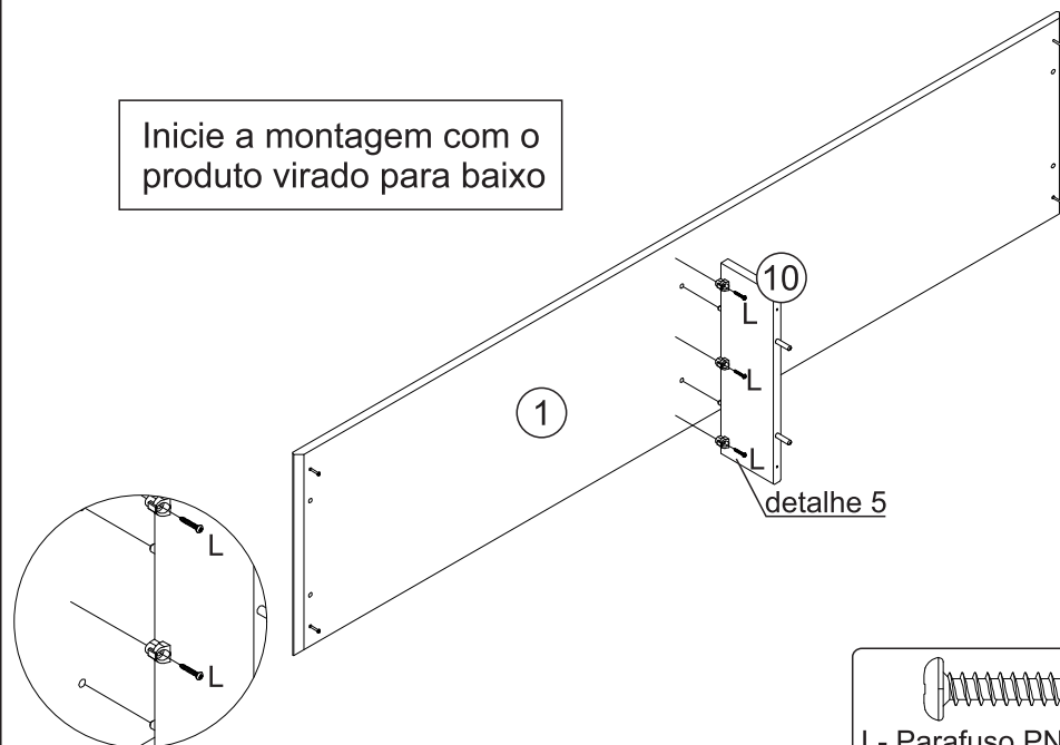
detalhe 5
