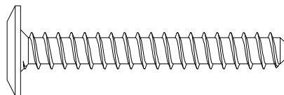
I- Parafuso estrutural ZP 7,0X50mm sx interno cab 17mm (5X) Cod 15892
