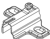
K- Calço H12 p/dobradiça 26mm (4X) Cod 54980
