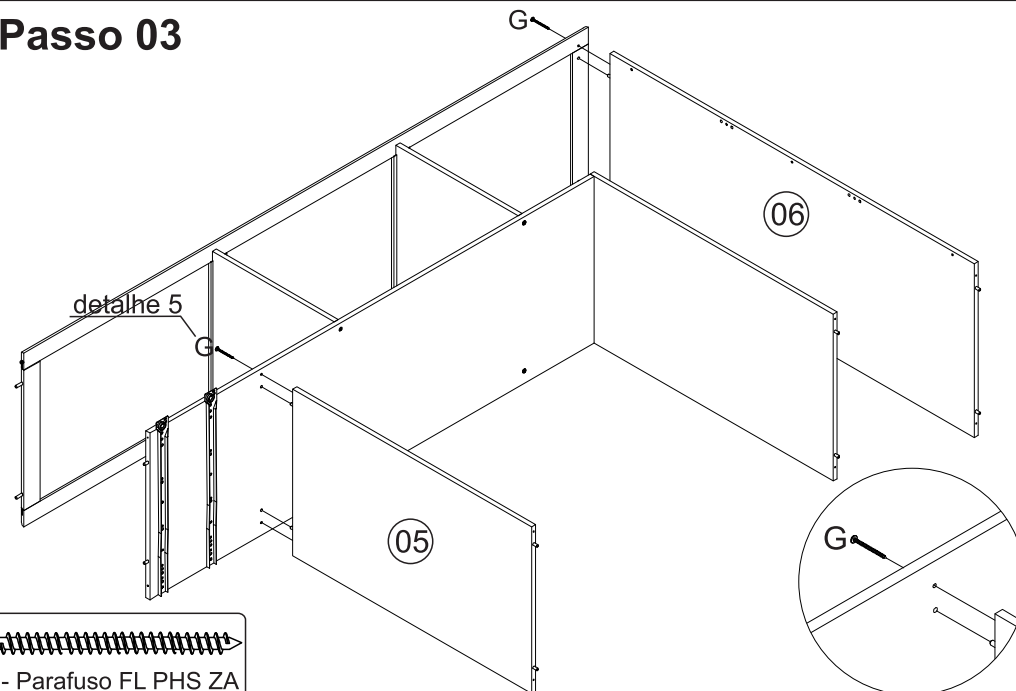
detalhe 5
