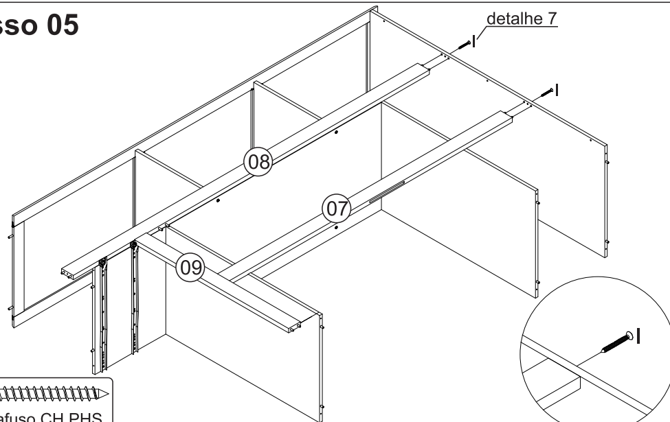
detalhe 7
