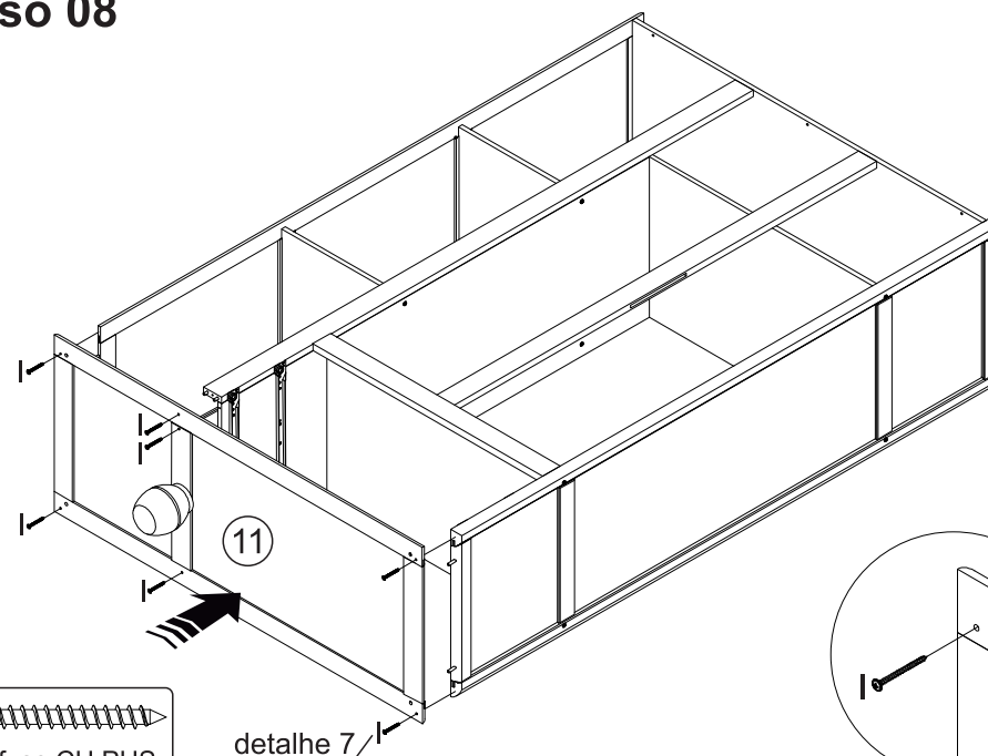
detalhe 7
