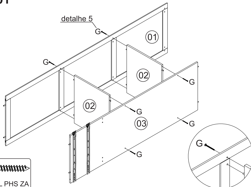
detalhe 5
